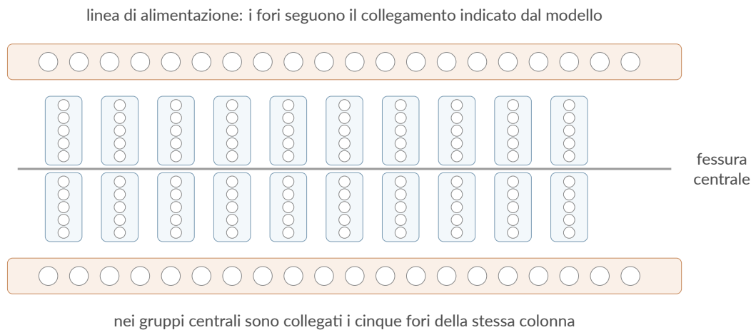
Figura A.6: Organizzazione tipica dei collegamenti interni di una breadboard. Prima dell'uso è opportuno verificare il modello disponibile in laboratorio.
